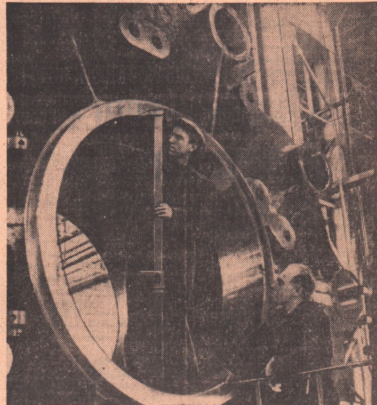
ЮЖУРАЛМАШЗАВОД. В первом механическом цехе предприятия идет расточка привода конвертора. Орчане изготавливают его по заказу челябинских металлургов.
