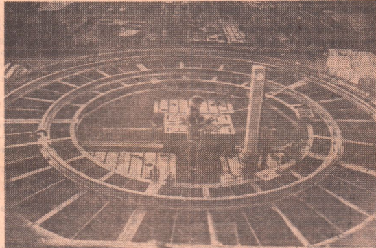
Южуралмашзавод. Кольцевая нагревательная печь для Орского завода по обработке цветных металлов.
