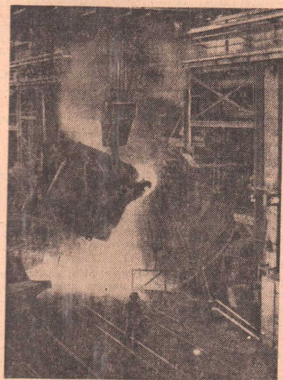
С МАРКОЙ «ЮУМЗ». КОНВЕРТОР В КОНВЕРТОРНОМ ЦЕХЕ НИЖНЕ-ТАГИЛЬСКОГО МЕТАЛЛУРГИЧЕСКОГО ЗАВОДА. Фото И. ГЕРГЕЛЯ.
