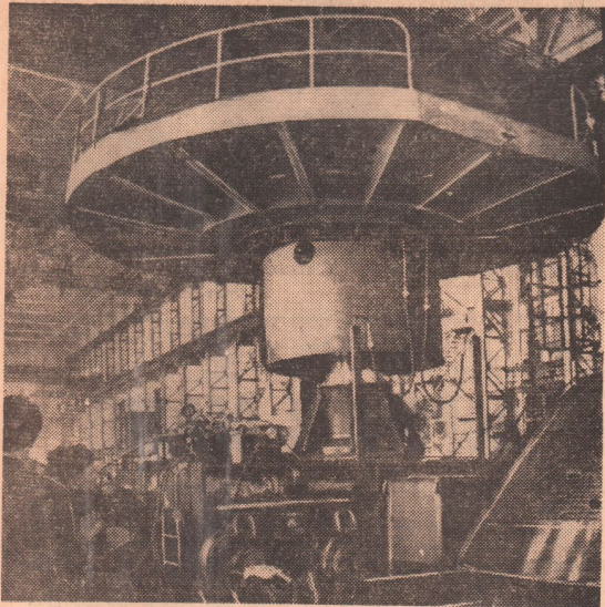
На Южуралмашзаводе закончены сборка и испытание домкратной гидравлической тележки для металлургов Финляндии.
