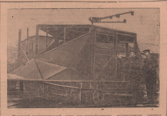
Московский экспериментальный завод сель-кохозяйственного машиностроения закончил сборку двух новых парниковых комбайнов, предназначенных для механизации парниковых горночашек, культивации и рыхления почвы, а также помп. Работает комбайн от электродвигателя. На снимке: подготовка нового комбайна к испытаниям.
