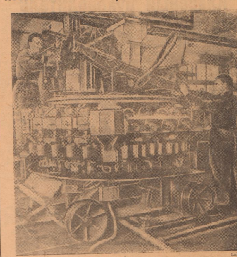
Коллектив московского завода «Стекломашин» создал и освоил выпуск для стекольной промышленности вакуумно-выдувного типа. Он представляет собой машину карусельного типа. Выдувка стекляной массы в форму производится посредством выдувных трубок, расположенных в форме параболы в каждой Секции. В свою очередь, вращается вокруг своей оси. Калибры распыленной стекляной массы подается в трубки вакуумным питателем. Во избежание перегрева форм и наборных головок вакуумного питателя они охлаждаются водой, циркулирующей по специальным каналам. Автомат «BC-24» заменяет ручной труд 180 стеклодувов. Его производительность — 20,000 стаканов в сутки.
